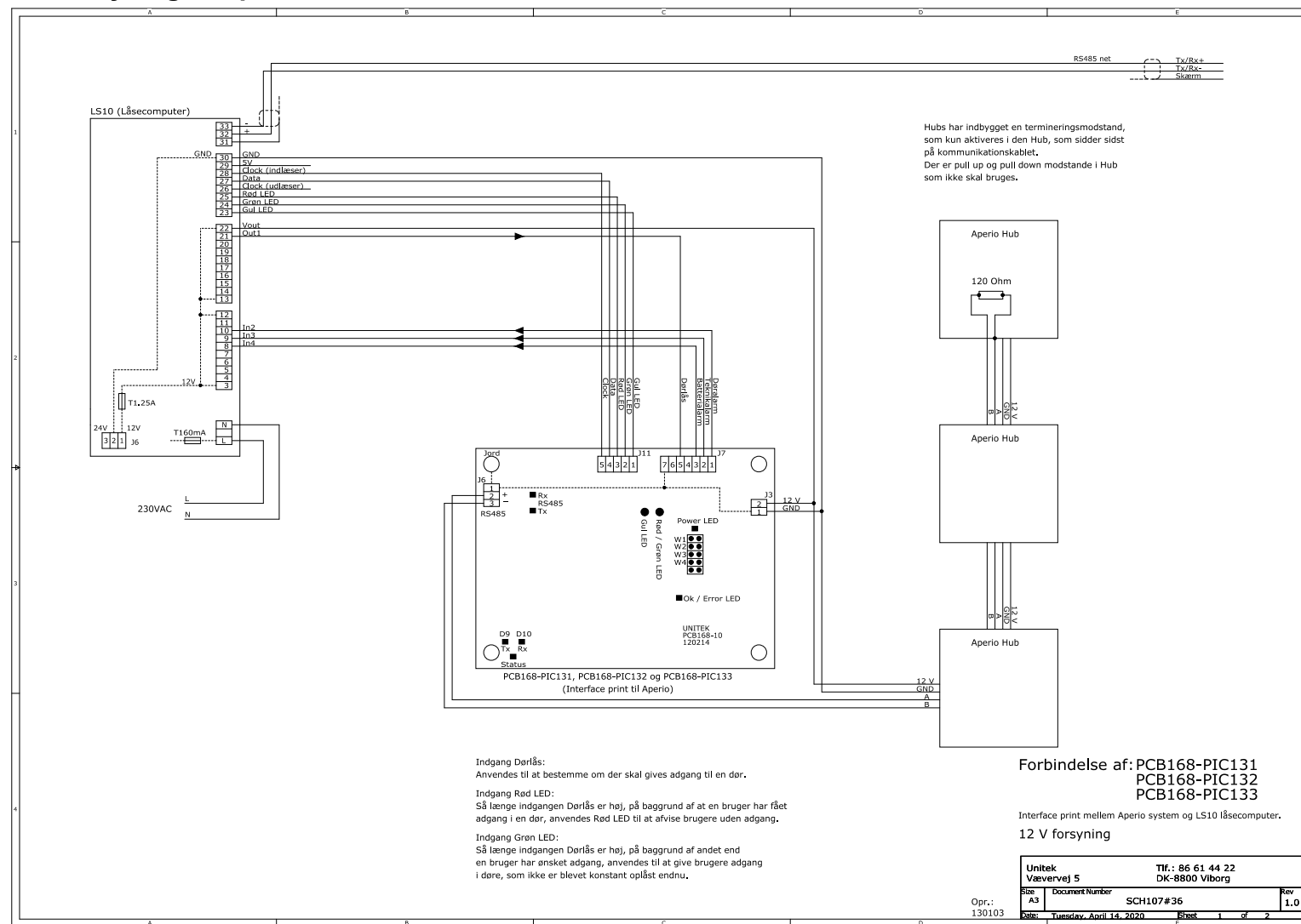
Figur 1. Tilslutning af PCB168-PIC131, PCB168-PIC132 og PCB168-PIC133
