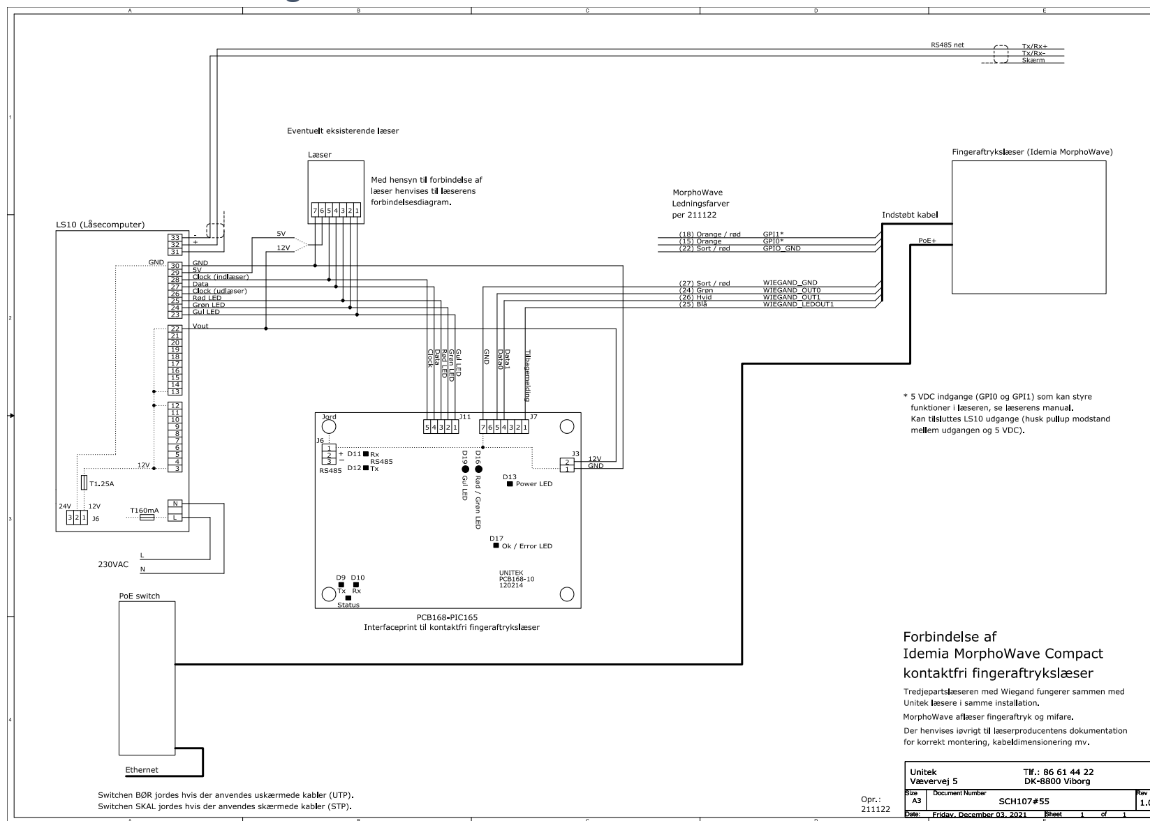
Figur 4. Tilslutning af PCB168-PIC165
