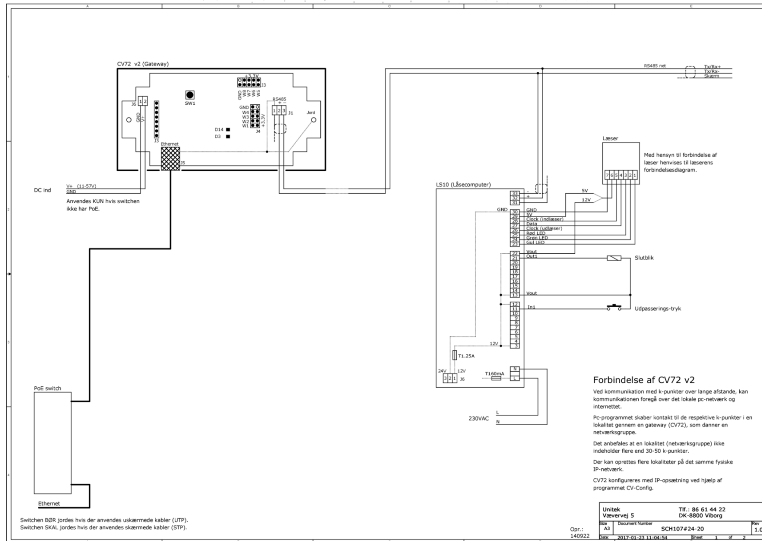
Figur 1. Tilslutning af CV72
