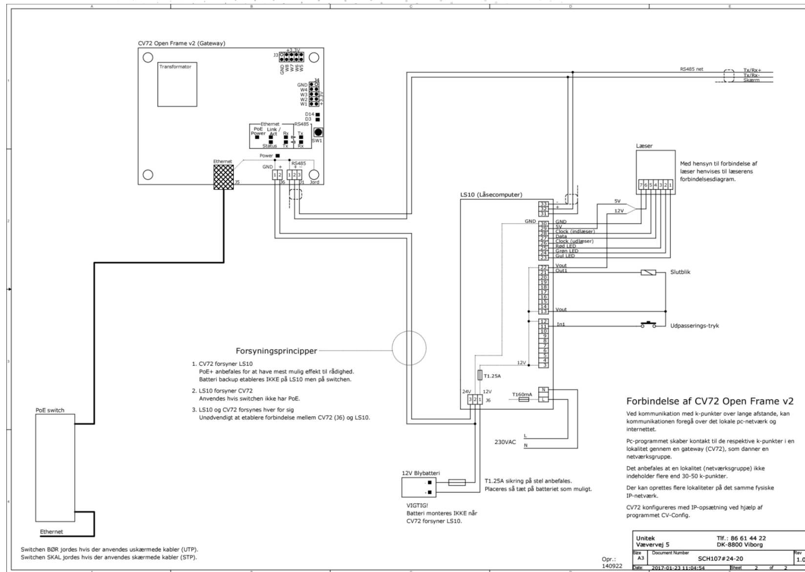
Figur 2. Tilslutning af CV72 Open Frame
