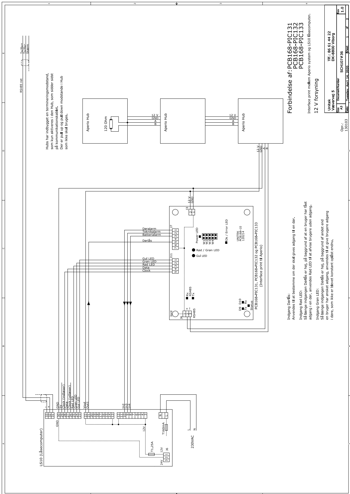
Figur 1. Tilslutning af PCB168-PIC131, PCB168-PIC132 og PCB168-PIC133
